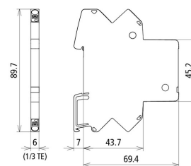
Dimensioni BCO CL2 BD HF 5
