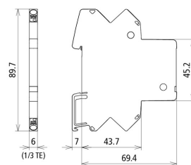
Dimensioni BCO CL2 BD 24
