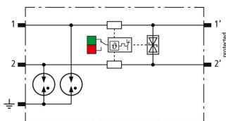
Schema di circuito basilare BCO ML2 BD HF 24
