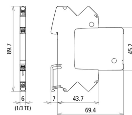
Dimensioni BCO ML2 BD 24
