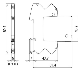
Dimensioni BCO ML2 BD 12
