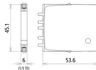
Dimensioni BCO MOD ML2 BE HF 24
