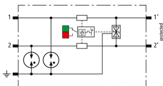
Schema di principio BCO MOD ML2 BE HF 5
