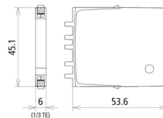
Dimensioni BCO MOD ML2 BE HF 5
