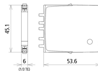
Dimensioni BCO MOD ML2 BD 48
