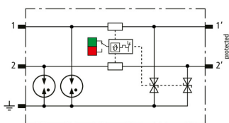
Schema di circuito basolare BCO MOD ML2 BE 180
