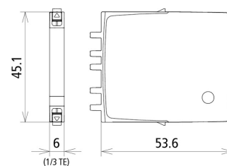
Dimensioni BCO MOD ML2 BE 180
