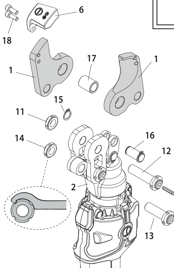
FIG. / BILD 3
