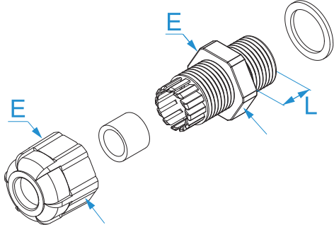
Disegno tecnico
