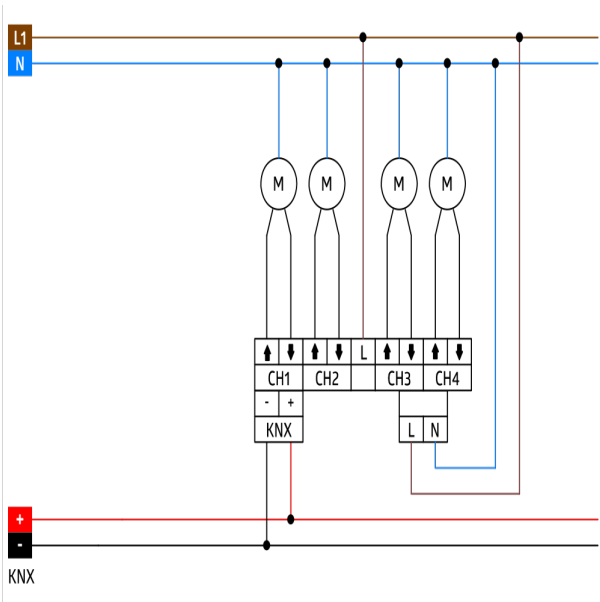
Schemi elettrici
