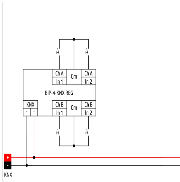
Schemi elettrici
