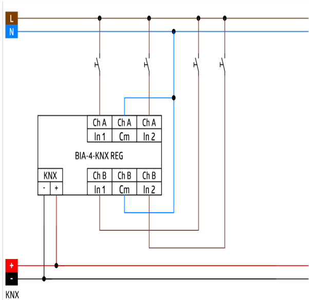
Schemi elettrici
