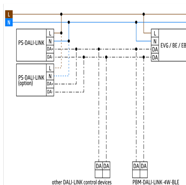
Schemi elettrici
