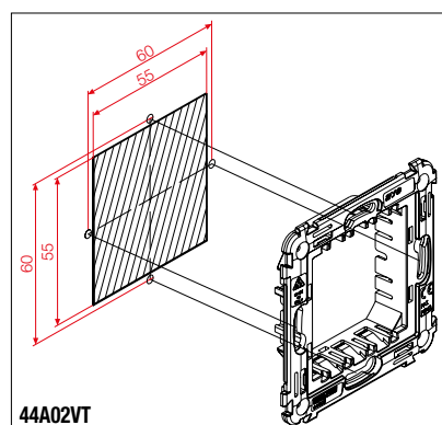
44A02 44A02SG 44A02VT
