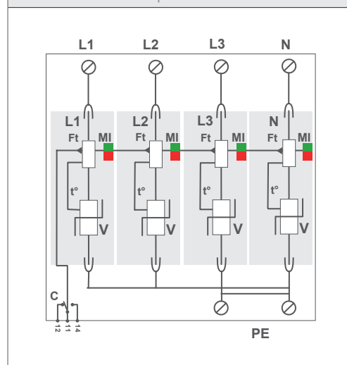
Schema di principio Principle scheme
