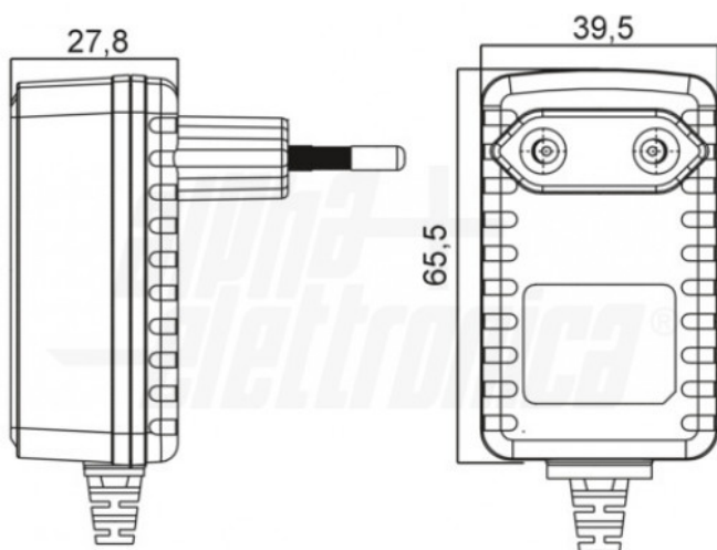
Dimensioni
