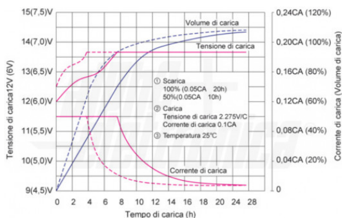
Curva di carica
