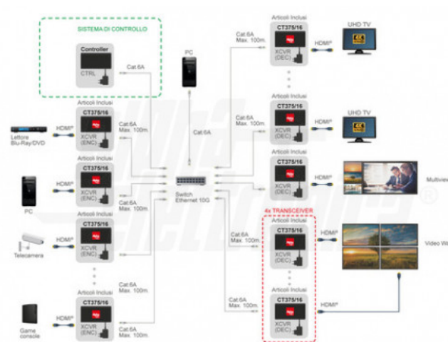
Collegamenti - Modalità 2
