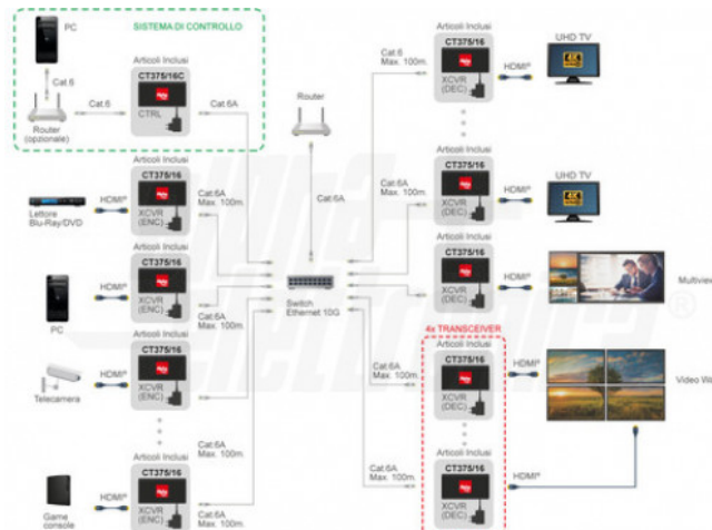
Collegamenti - Modalità 2
