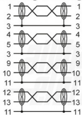
DVI Plug DVI Plug
