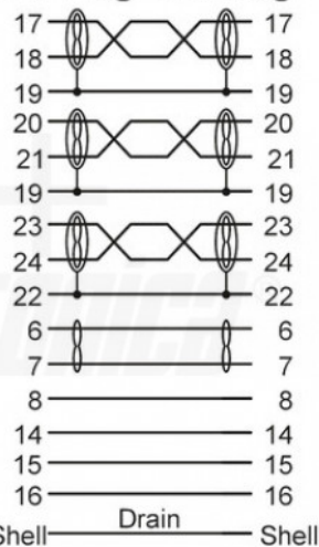
DVI Plug DVI Plug
