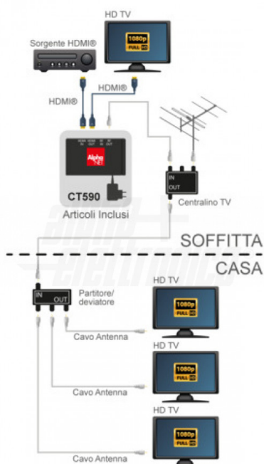
Installazione su ingresso antenna inutilizzato
