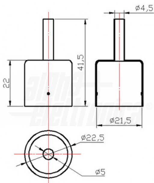
Dimensioni ugello
