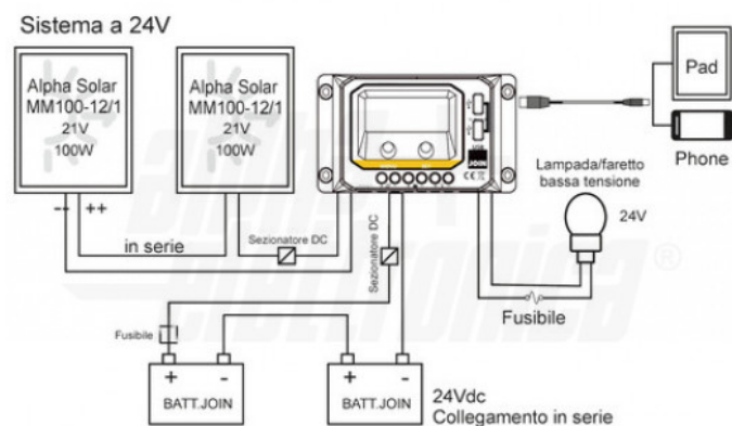
Collegamenti impianto a 24Vdc
