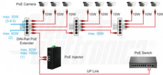
Modalità cascata
