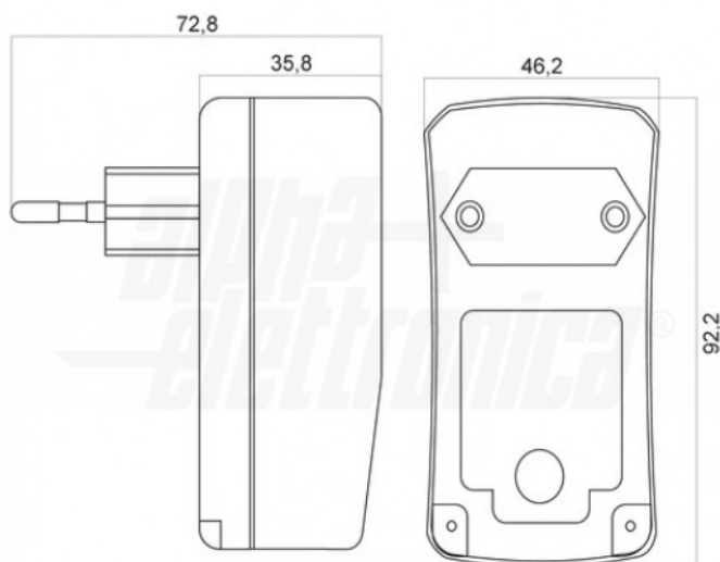
Dimensioni
