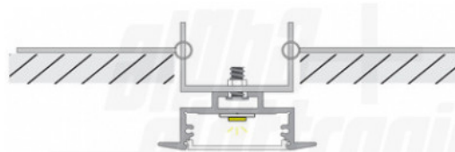
Installazione
