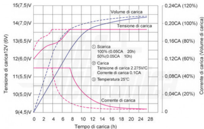
Curva di carica
