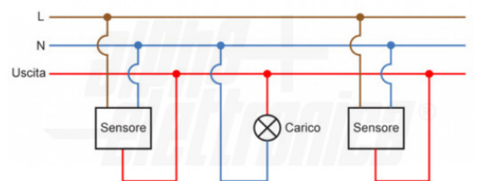
Collegamento in parallelo
