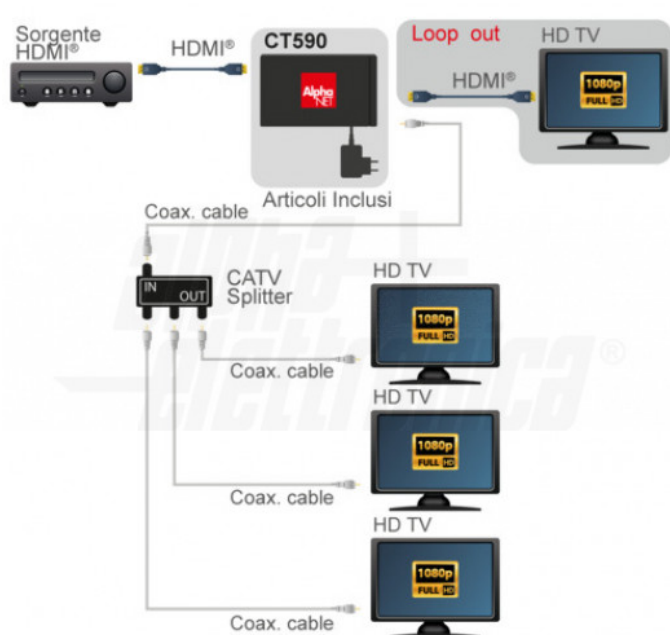
Installazione su ingresso antenna inutilizzato
