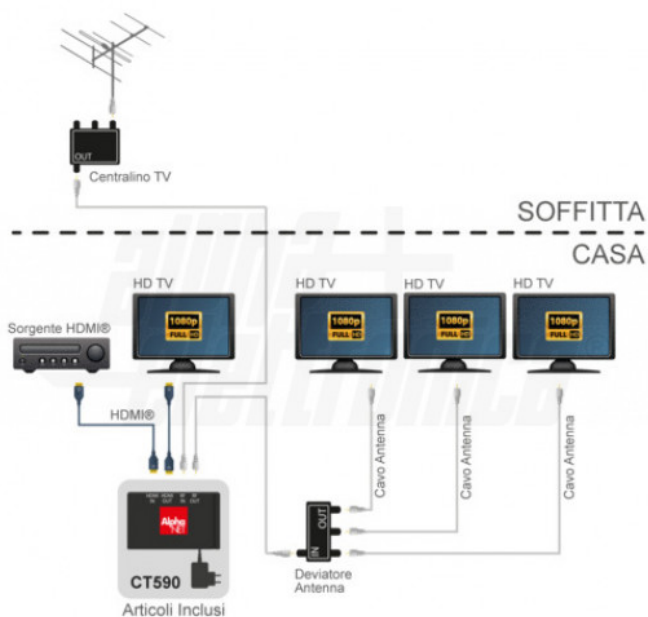
Installazione con modulatore in casa
