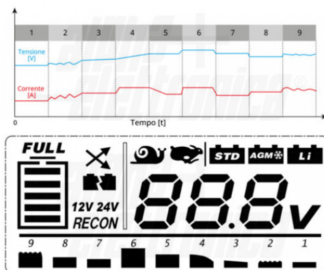
Curva di ricarica a 9 fasi smart
